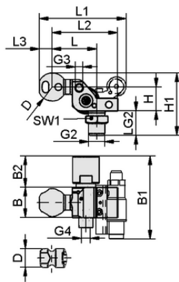
Dati di costruzione HT-SG A2 I 10 31 NPT3/8-AG AB
