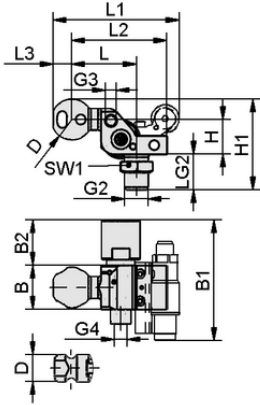
Tasarım verileri HT-SG A5 I 10 31 NPT3/8-AG AB
