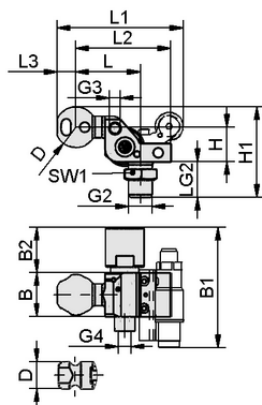
デザインデータ HT-SG A3 I 10 31 NPT3/8-AG AB
