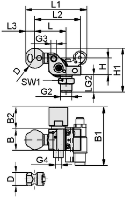
Tasarım verileri HT-SG A2 I 10 31 G3/8-AG AB
