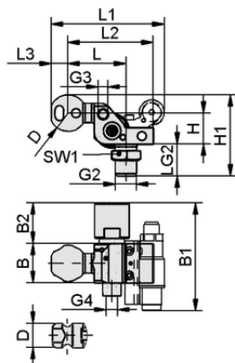
Design data HT-SG A2 I 10 31 G3/8-AG AB
