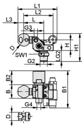
デザインデータ HT-SG A2 I 10 31 G3/8-AG AB
