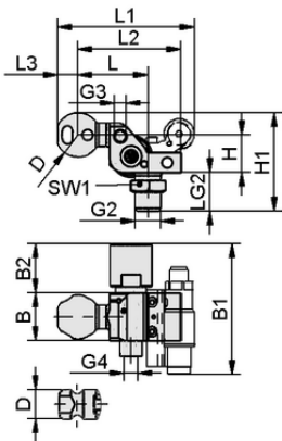
Design data HT-SG A5 I 10 31 G3/8-AG AB
