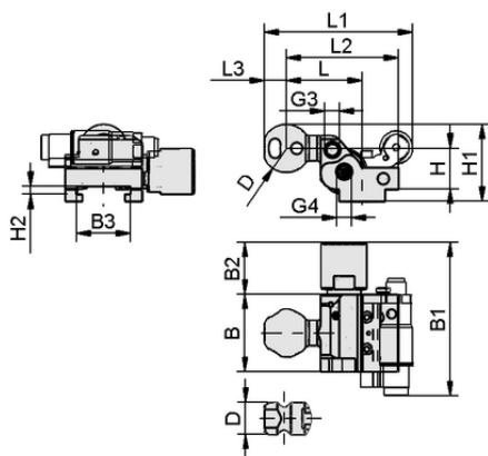
Design data HT-SG A2 I 10 46 RA AB
