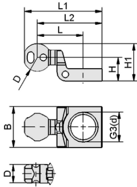
Tasarım verileri HT-FST A2 42 M30x1.5
