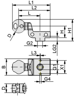
Tasarım verileri HT-SG A2 E 35 M16x1.5-IG
