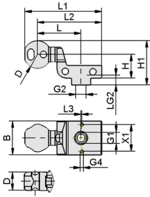
Tasarım verileri HT-SG A5 E 35 M14x1.5-IG
