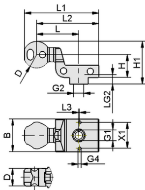
Dati di costruzione HT-SG A3 E 35 M14x1.5-IG
