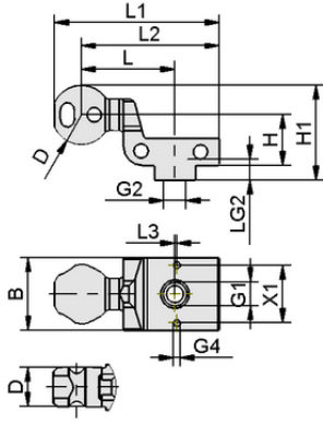
Tasarım verileri HT-SG A2 E 35 M10-IG
