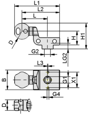
Tasarım verileri HT-SG A3 E 35 M10-IG
