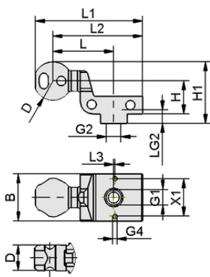
Dati di costruzione HT-SG A3 E 35 M10-IG
