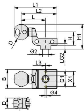
Design data HT-SG A2 E 35 G1/4-IG
