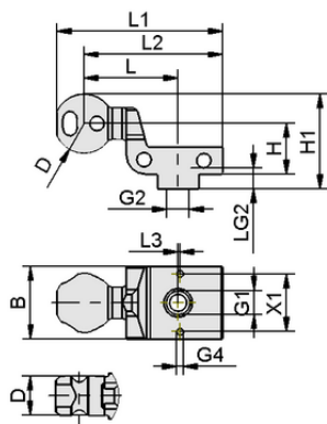
デザインデータ HT-SG A5 E 35 G1/4-IG
