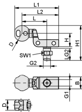
Dati di costruzione HT-SG A2 22 NPT3/8-AG
