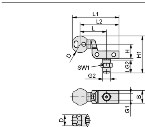
デザインデータ HT-SG A2 22 NPT3/8-AG
