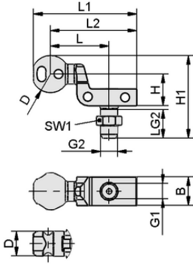
Tasarım verileri HT-SG A3 22 NPT3/8-AG
