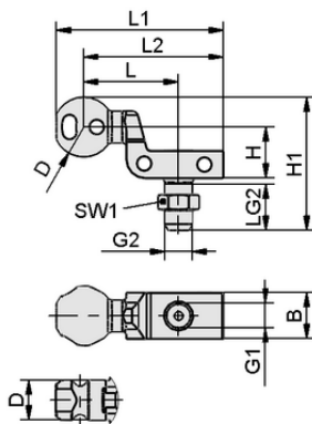
Dati di costruzione HT-SG A2 22 G3/8-AG
