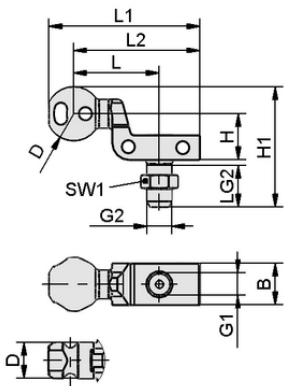
Design data HT-SG A5 22 G3/8-AG
