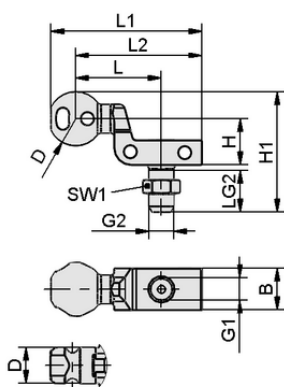
Dati di costruzione HT-SG A2 22 NPT1/4-AG
