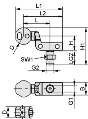
Dati di costruzione HT-SG A5 22 NPT1/4-AG
