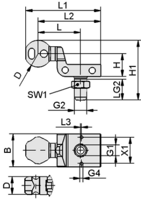
Tasarım verileri HT-SG A2 E 35 NPT3/8-AG
