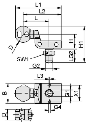
Données de construction HT-SG A5 E 35 NPT3/8-AG
