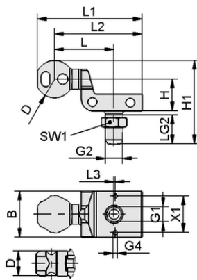
Konstruktionsdaten HT-SG A2 E 35 G3/8-AG
