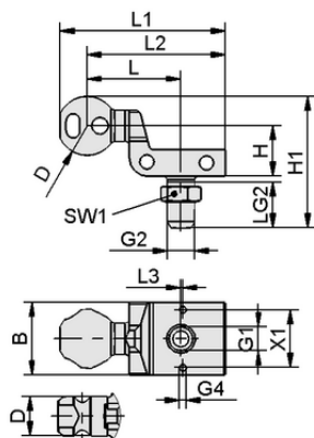
デザインデータ HT-SG A2 E 35 G3/8-AG
