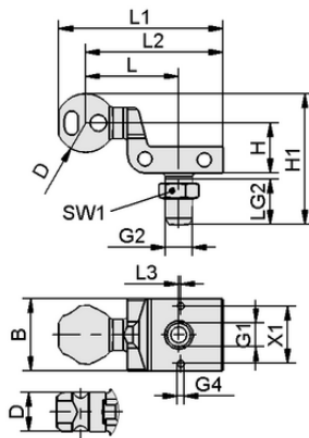
Dati di costruzione HT-SG A2 E 35 G3/8-AG
