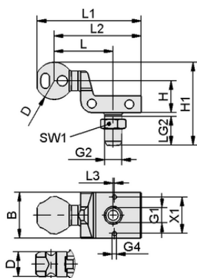
Dati di costruzione HT-SG A5 E 35 G3/8-AG
