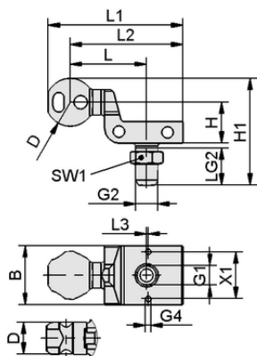
デザインデータ HT-SG A5 E 35 G3/8-AG
