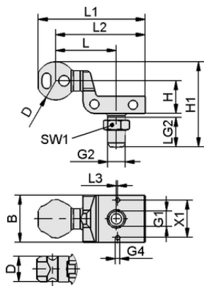
Design data HT-SG A3 E 35 NPT3/8-AG
