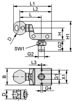
デザインデータ HT-SG A2 E 35 NPT1/4-AG
