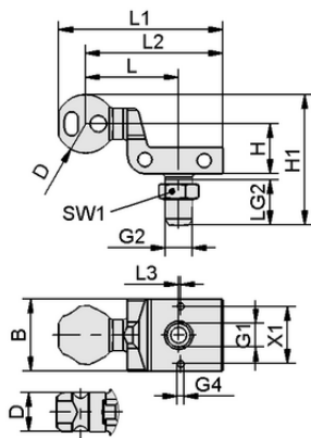
Design data HT-SG A5 E 35 NPT1/4-AG
