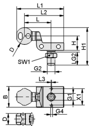
Données de construction HT-SG A5 E 35 NPT1/4-AG
