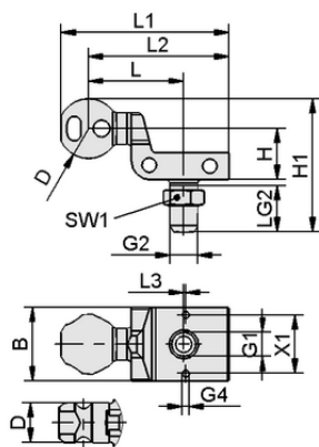
デザインデータ HT-SG A3 E 35 NPT1/4-AG
