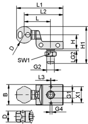
Design data HT-SG A3 E 35 NPT1/4-AG
