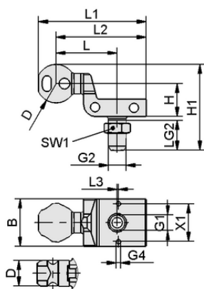
Données de construction HT-SG A2 E 35 G1/4-AG
