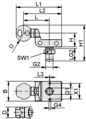
デザインデータ HT-SG A2 E 35 G1/4-AG
