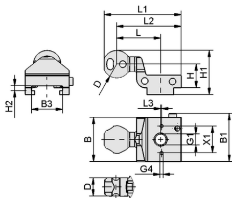
デザインデータ HT-SG A2 E 46 RA
