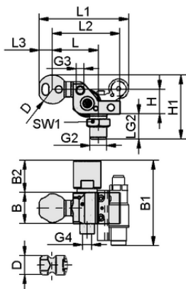
Design data HT-SG A3 I 10 31 G3/8-AG AB
