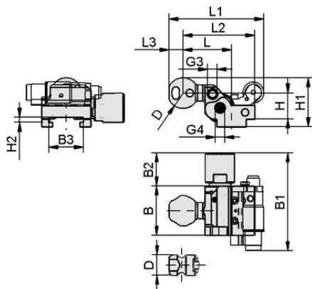
Design data HT-SG A3 I 10 46 RA AB
