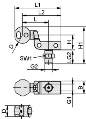
Design data HT-SG A3 22 G3/8-AG
