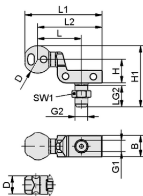
Dati di costruzione HT-SG A3 22 G1/4-AG
