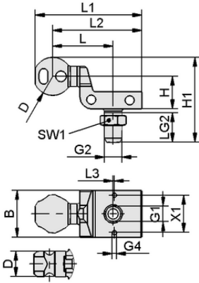
Tasarım verileri HT-SG A3 E 35 G3/8-AG
