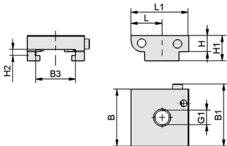
Konstruktionsdaten HT-SG 46 RA
