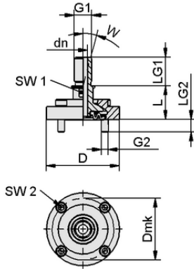
Tasarım verileri FLK-HD G1/4-IG
