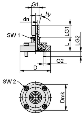
デザインデータ FLK-HD G1/4-IG
