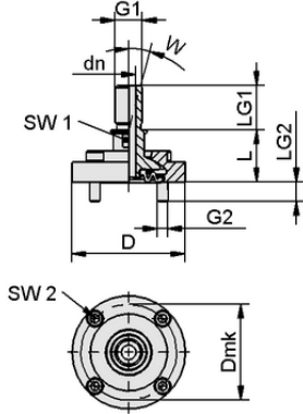
Tasarım verileri FLK-HD G3/8-AG
