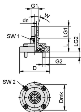
Datos de diseño FLK-HD G3/8-AG
